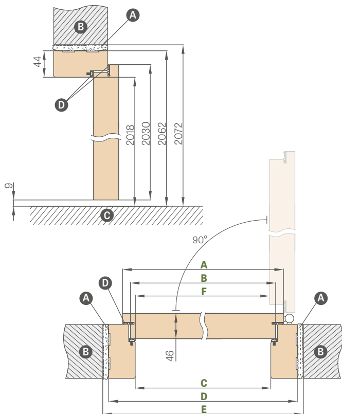
HERSE SET FIX AJTÓTOK KERESZTMETSZETE
